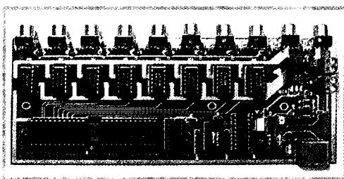
La scheda AVS8 per la commutazione di segnali audio/video.
