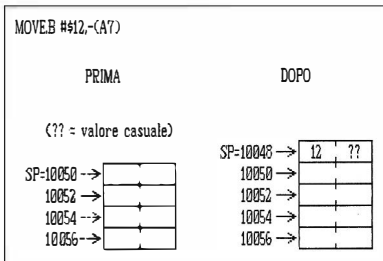
Fig. 3 push di un byte...
