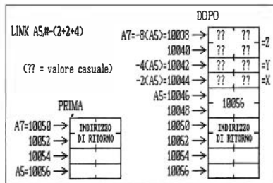
Fig. 4 Allocazione di 8 byte...
