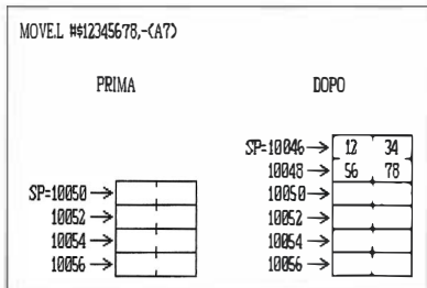
Fig. 1 push di una long word
