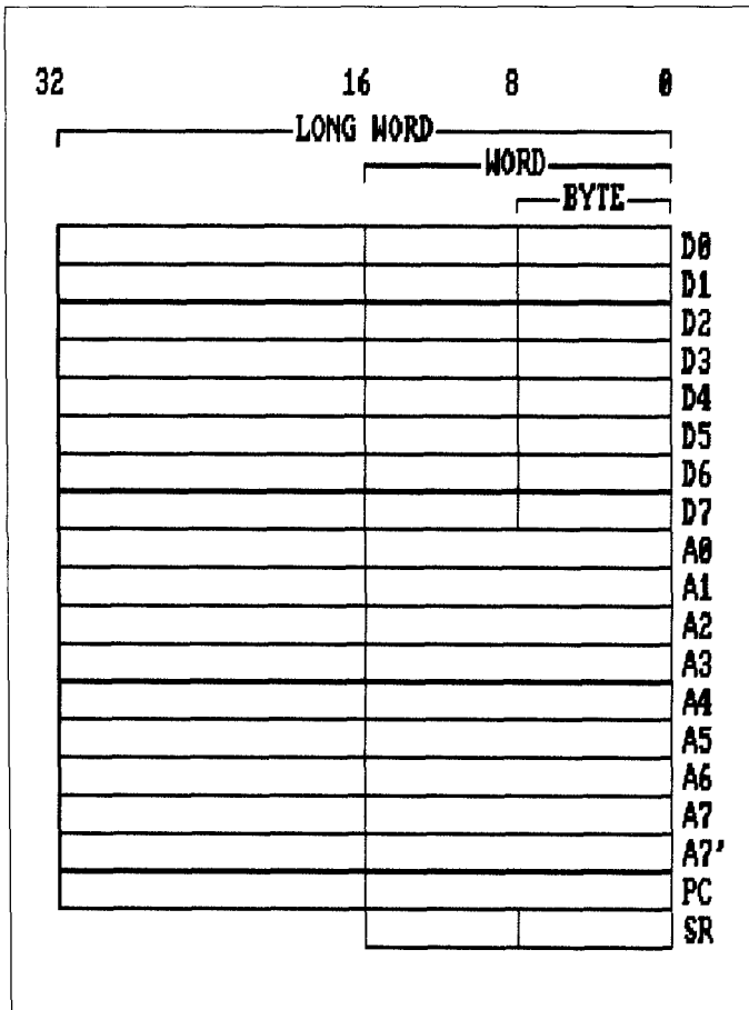
Schema dei registri del processore.
