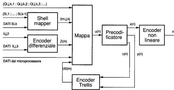
Schema a blocchi del modulatore V34. La modulazione V34 è molto complessa.
